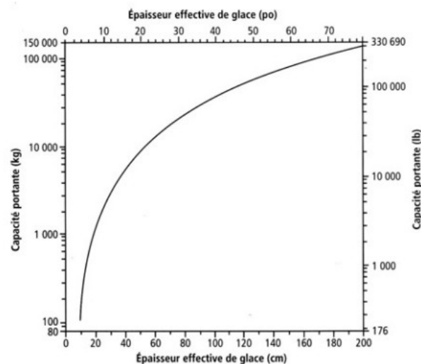
ILLUSTRATION 9 Courbe de la capacité portante en fonction de l'épaisseur effective
